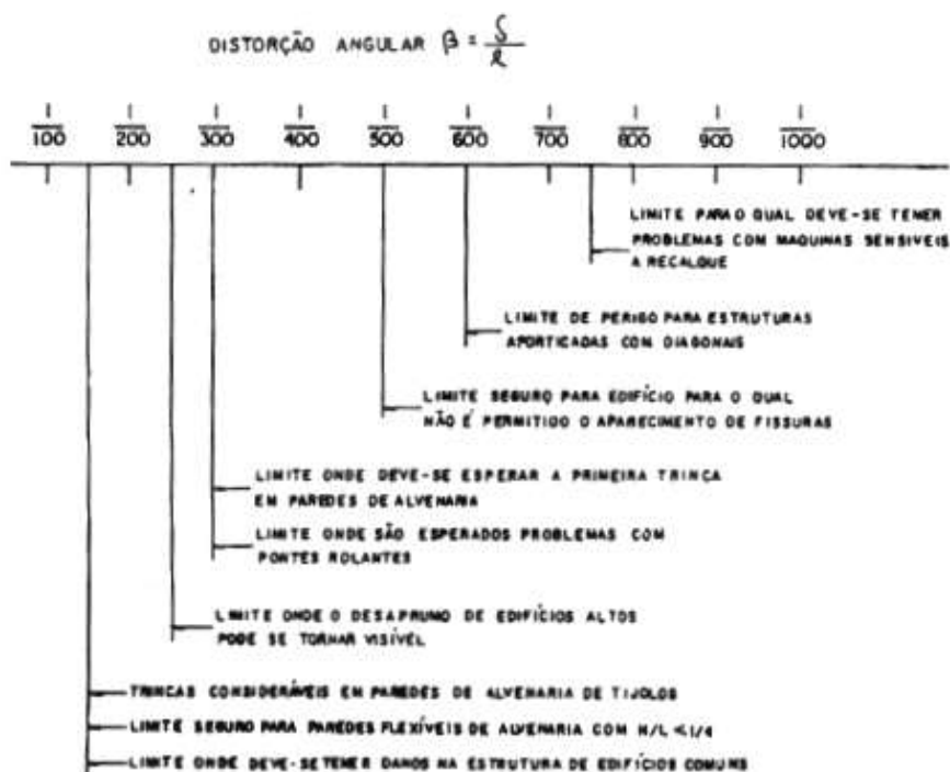
Figura 4. Valores admissíveis de distorção angular. (Bjerrum, 1963 apud Teixeira e Godoy, 1996)
