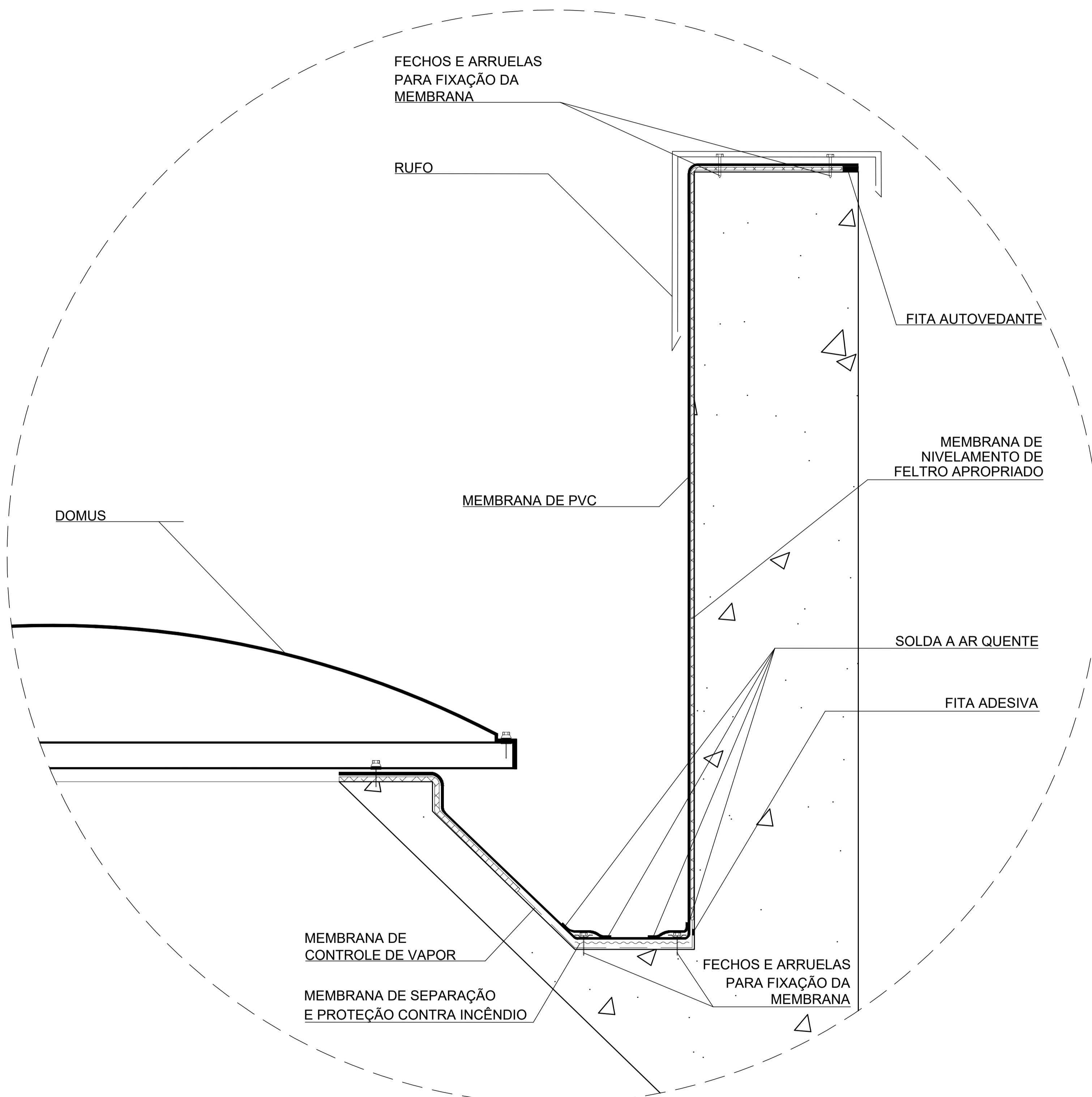
DETALHE 04 - ARREMATE DOMUS E RUFOS ESCALA 1:5
